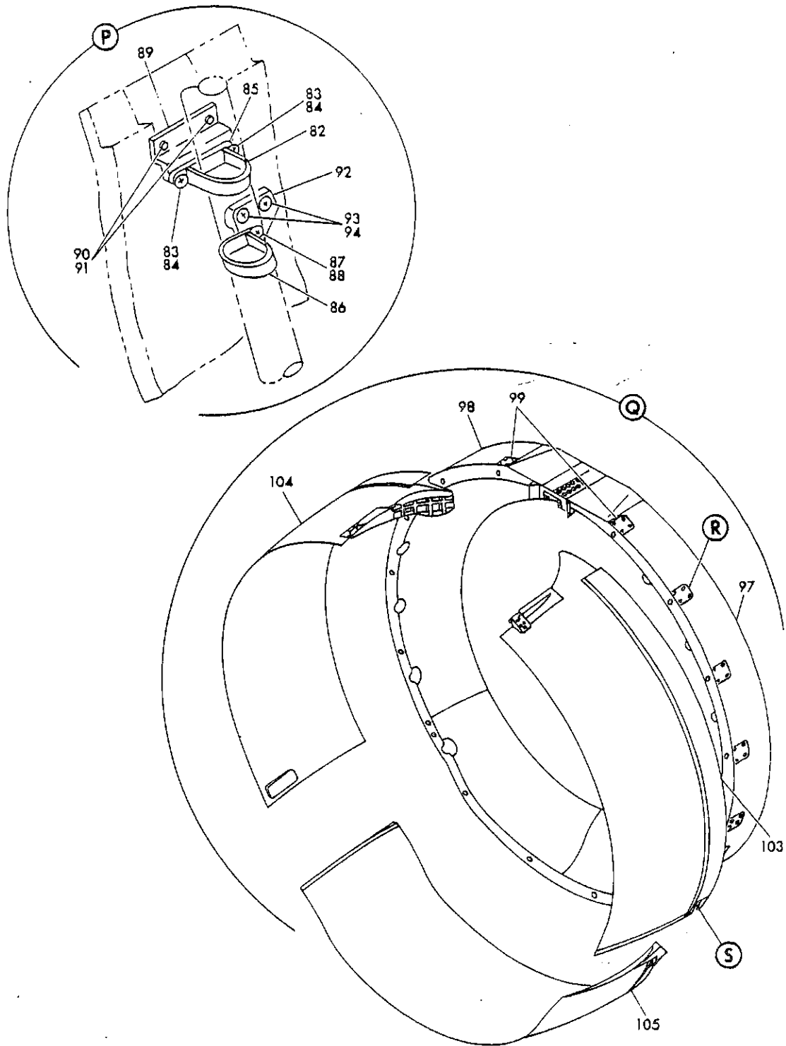
FIGURE 1. FAN REVERSER INSTL, FAN ENGINE (SHEET 5)
