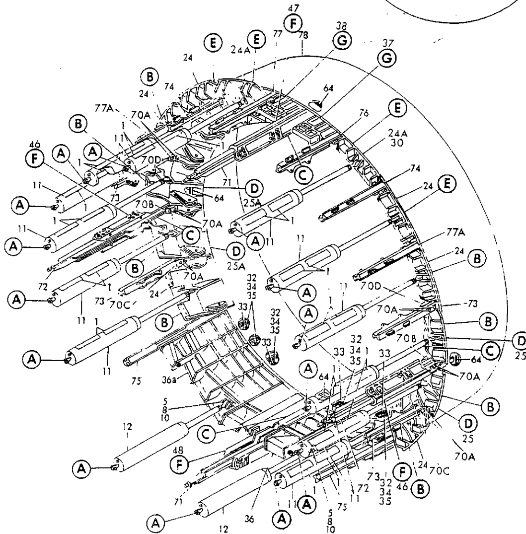
FIGURE 1B. FAN REVERSER INSTL. FAN ENGINE (SHEET 1)
