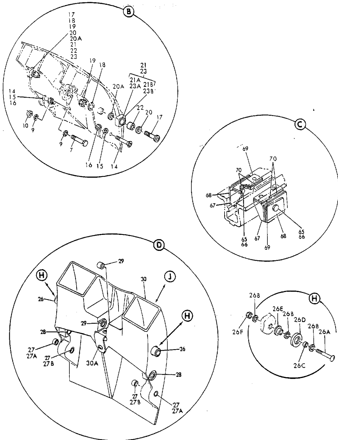
FIGURE 18. FAN REVERSER INSTL, FAN ENGINE (SHEET 2)
